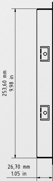
Unterputzgehäuse
